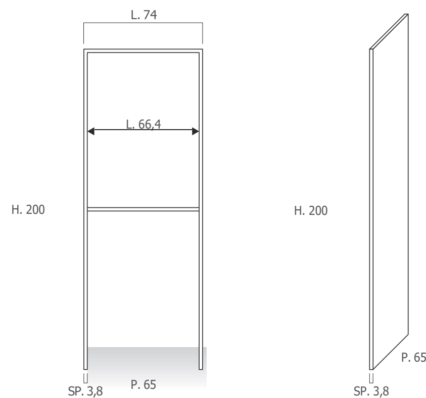
Colonna portalavatrice asciugatrice H. 200 - P. 65
