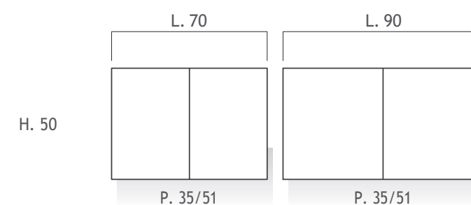
Basi sospese portalavabo 2 ante H. 50
