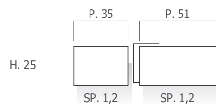
Fianchi terminali H. 25
