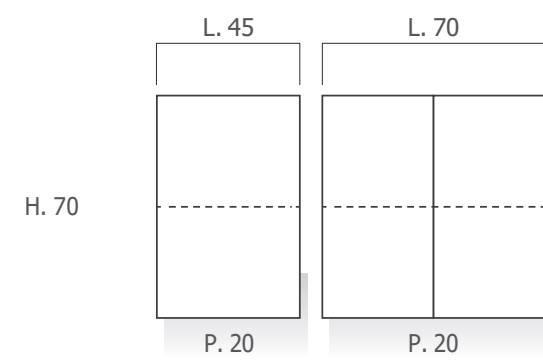
Pensili lavanderia 1 e 2 ante H. 70 - P. 20
