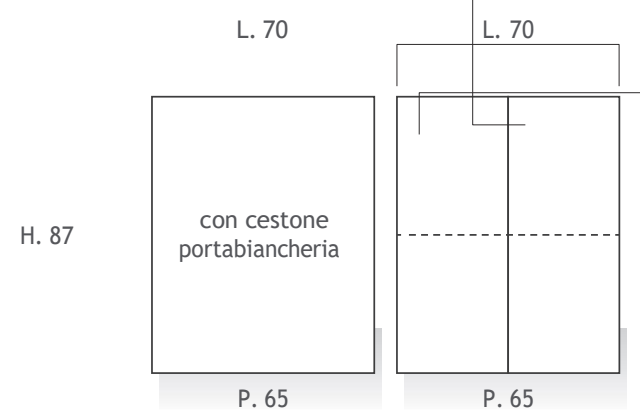
Basi lavella 1 e 2 ante H. 87 - P. 65
